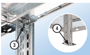
Fachbodenträger (3), Klemmfuß (4)
